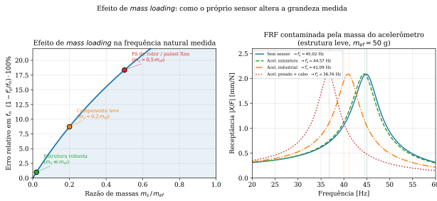
Figura 7: Efeito de mass loading. Fonte: O autor.
